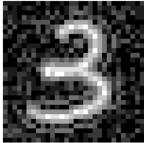
Nucleation model: VarHárom4
